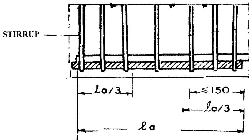
Fig. 8. Longitudinal section
