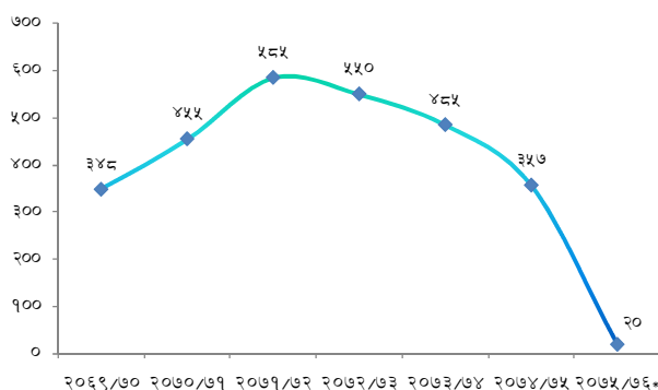
चार्ट १०(क): विद्युत माग र आपूर्ति बीचको अन्तर (मेगावाटमा)
