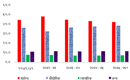
चार्ट १०(ग): क्षेत्रगत विद्युत खपत (प्रतिशतमा)
