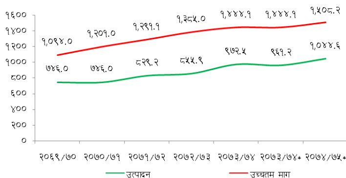
चार्ट १० (ख) : विद्युत माग र आपूर्ति बीचको अन्तर (मेगावाटमा)
