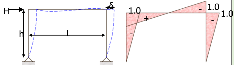
Case I: No brace
