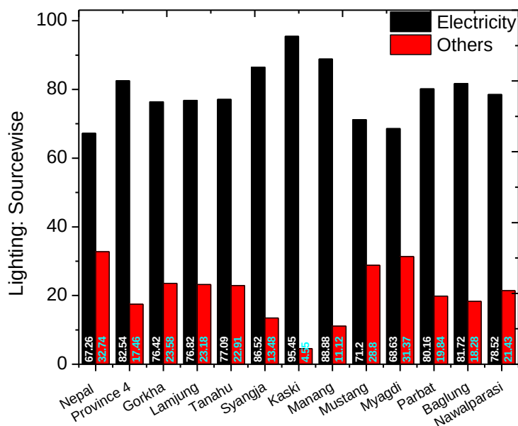
चित्र नं. ७.१ जिल्लागत घरहरू उज्यालो बनाउन प्रयोग विद्युत र अन्य ऊर्जा
